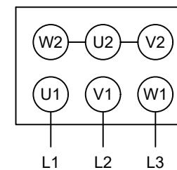
CABLAGE DU MOTEUR EN ETOILE
